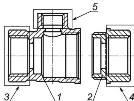
1, 2 — полукорпуса; 3, 4 — присоединительные концы; 5 — горловина
