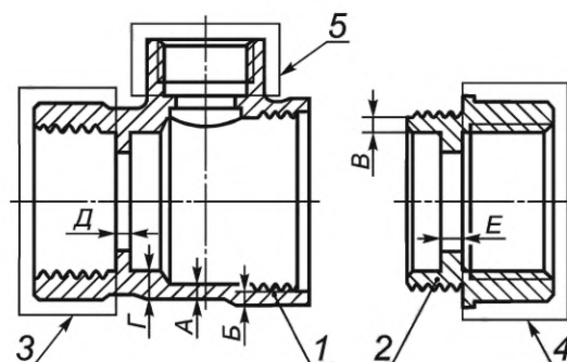
1, 2 — полукопруса; 3, 4 — присоединительные концы; 5 — горловина; А, В, С, Д, Е — места измерения толщины стенки корпуса крана
